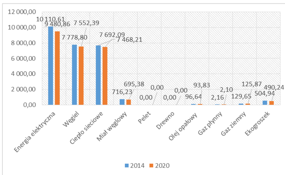
Wykres 27. Zmiana emisji CO 2 w perspektywie do 2020 r. [MgCO 2 ]
