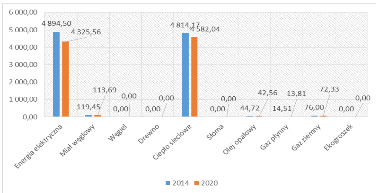
Wykres 23. Zmiana emisji CO 2 w perspektywie do 2020 r. [MgCO 2 ]
