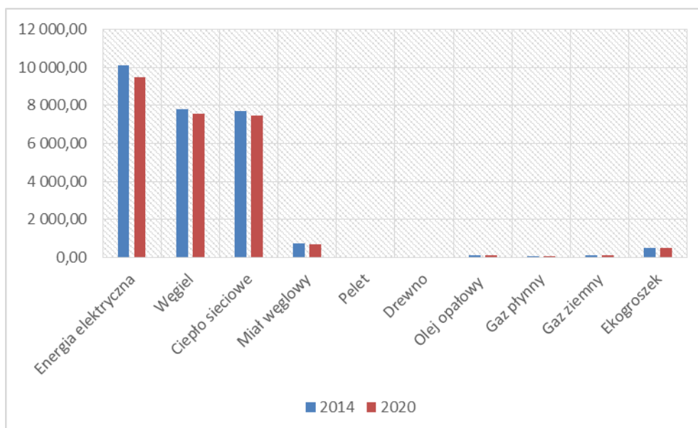
Wykres 10. Zmiana emisji CO 2 w budynkach mieszkalnych w perspektywie 2014-2020 [Mg CO 2 ]
