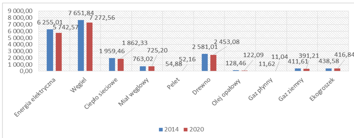
Wykres 29. Zmiana zużycia paliw pierwotnych i nośników energii w perspektywie do 2020 r. [MWh]
