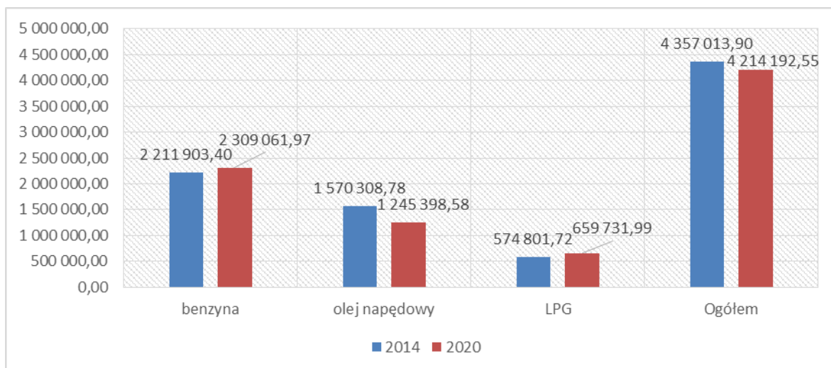
Wykres 33. Zmiana zużycia paliw pierwotnych i nośników energii w perspektywie do 2020 r. [t]
