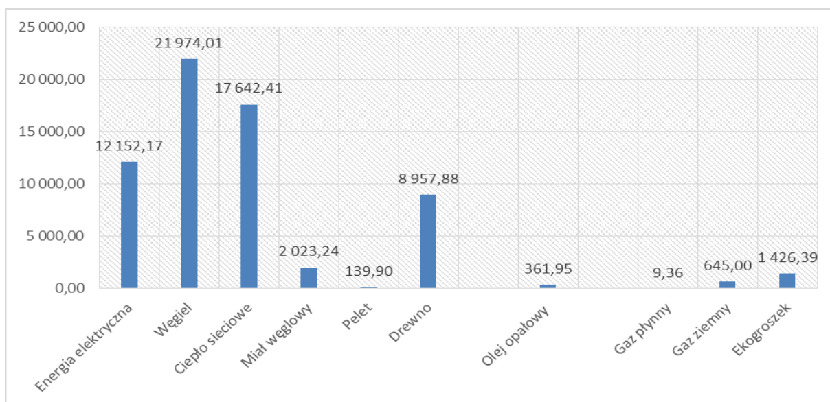
Wykres 24. Zużycie energii elektrycznej oraz paliw pierwotnych i nośników energii w 2014 r. [MWh]
