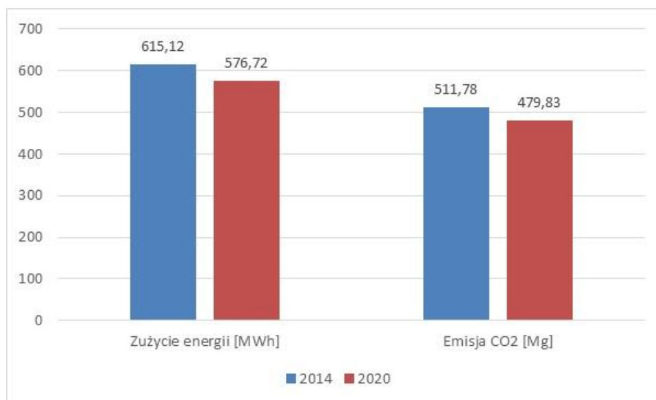
Wykres 18. Zużycie energii oraz emisja CO 2 związana z oświetleniem ulicznym
