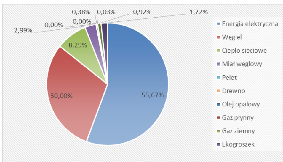
Wykres 12. Emisja CO 2 w sektorze przedsiębiorstw w roku 2014 [%]
